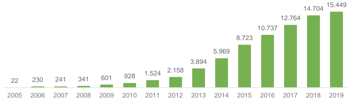
Evolução Histórica da Capacidade Instalada de Energia Eólica no Brasil (MW)
